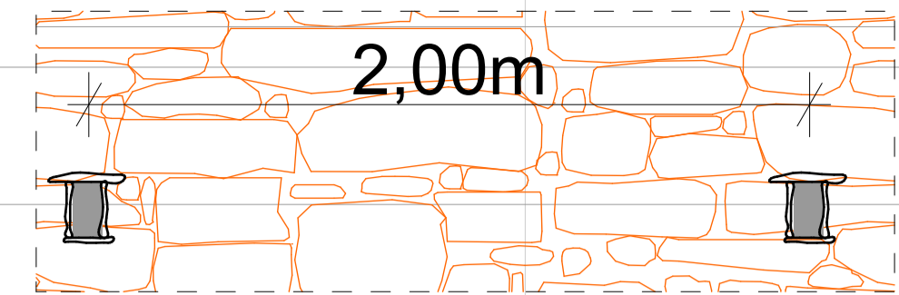
Detaliu D1 - 1:20
